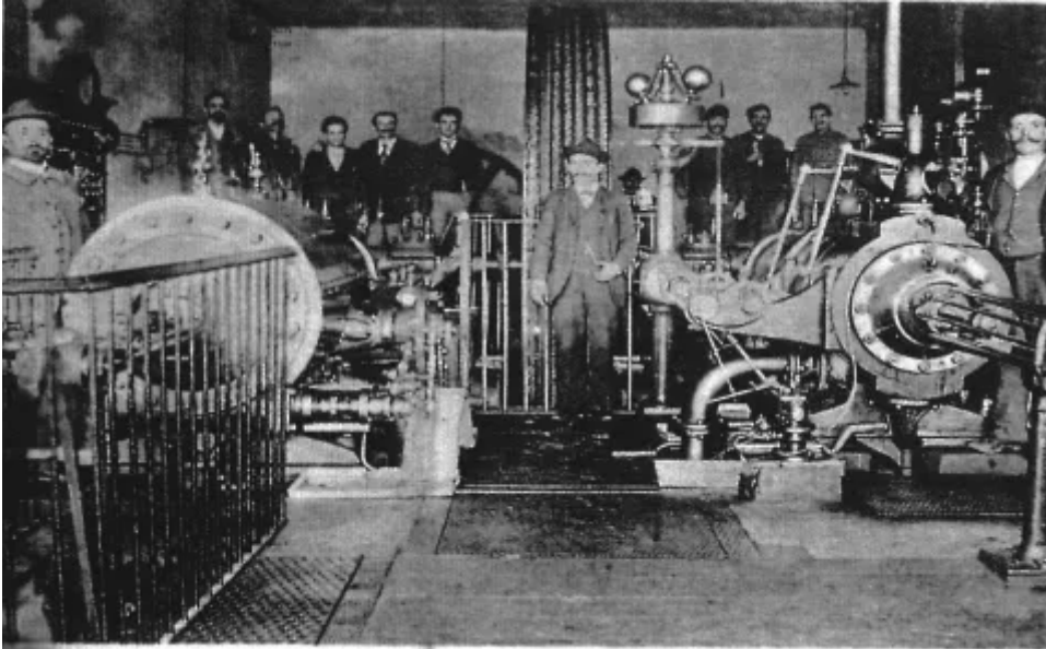
Dampfsäge in Sadova bei Kimpolung.
